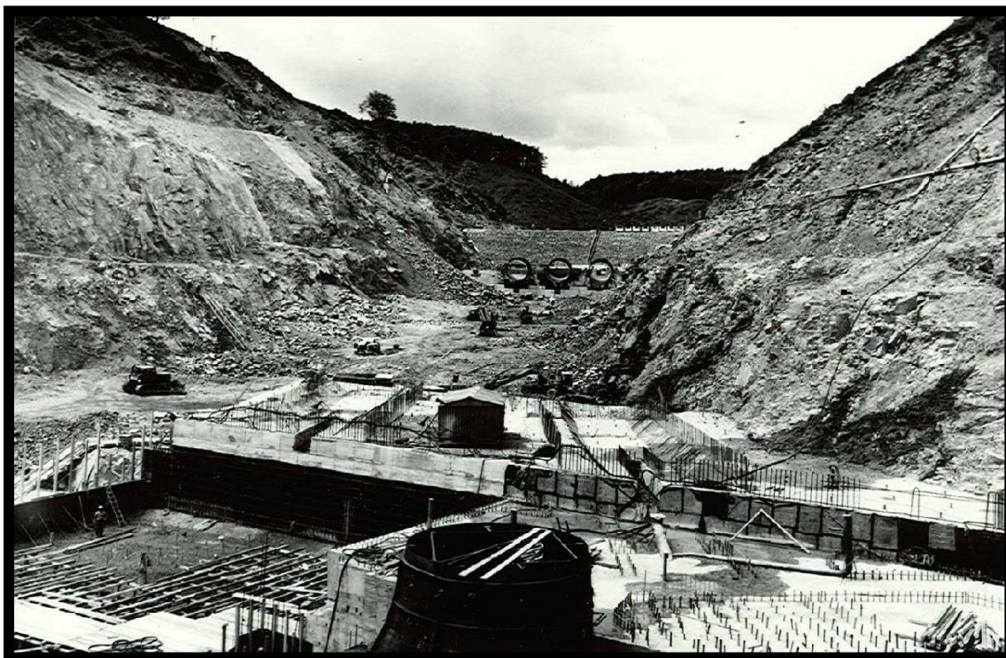
Obr. 1 Uložení savky č.1 – 2.9.1975
