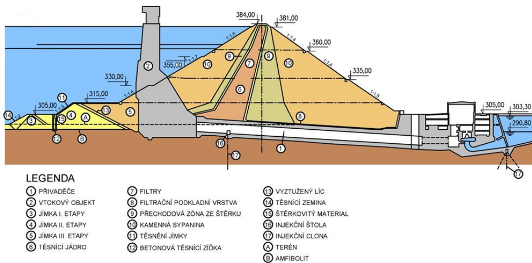
Obr. 5 Podélný řez VD Dalešice [3]
