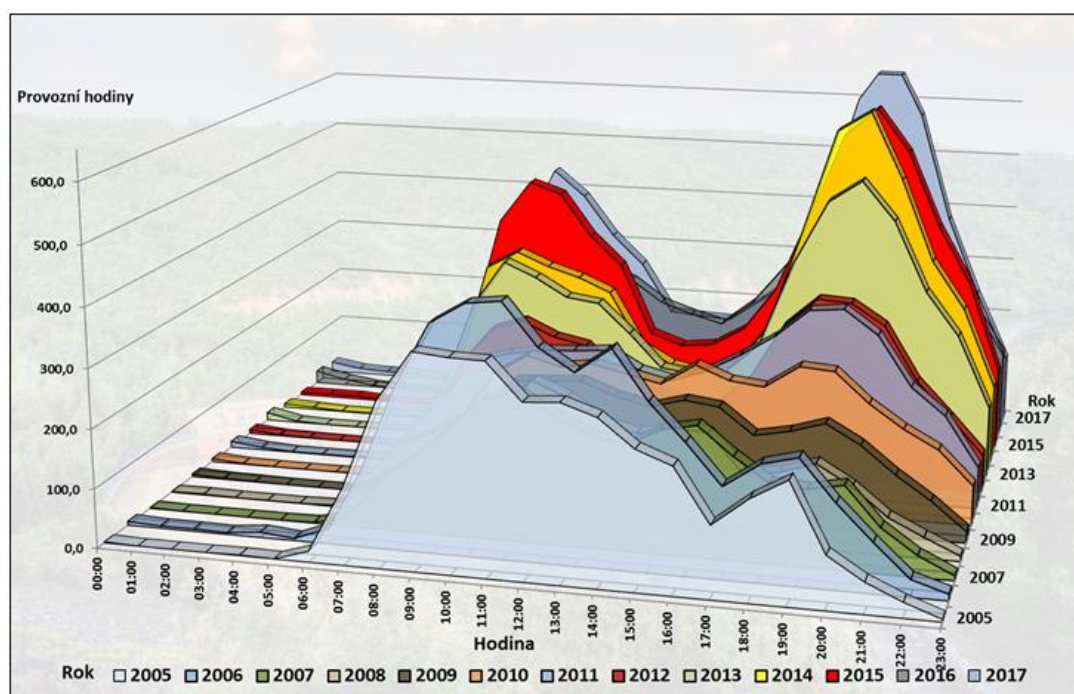
Graf 4 - Přehled provozních hodin turbínového provozu během dne. [8]
