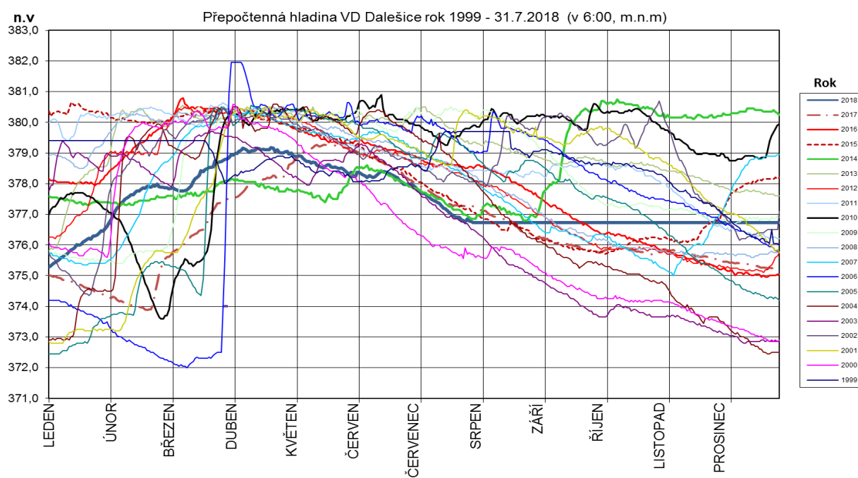
Graf 6 – Průběh hladin VDD 1999 – 2017 [10]
