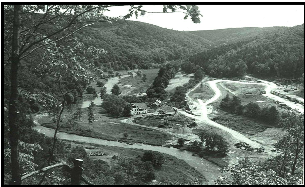
Zahájení stavby – 1971- pohled z hráze na Slavětický mlýn
