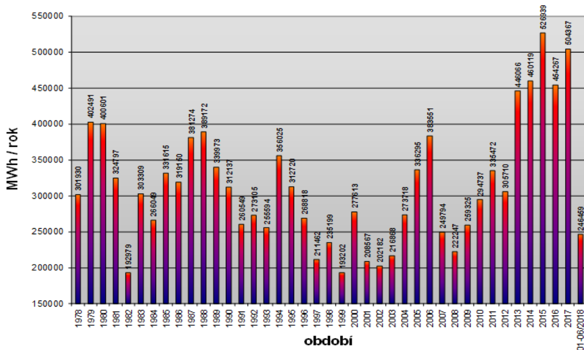
Graf 1 Výroba elektrárny (MWh) od uvedení do provozu do první poloviny roku 2018 [5]
