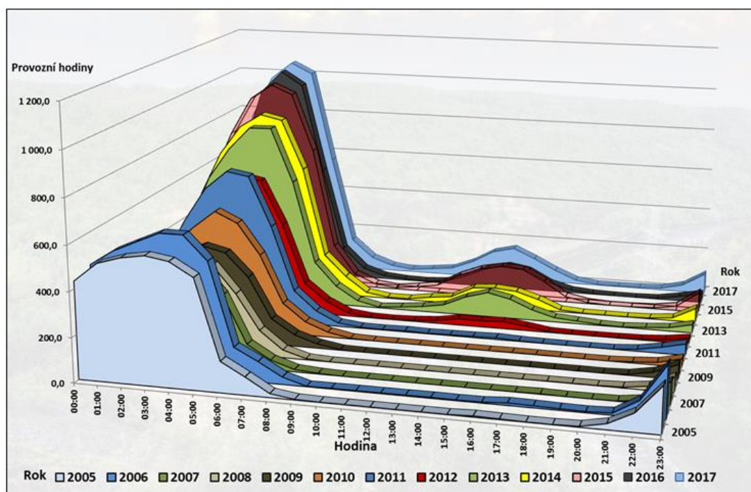
Graf 5 Přehled provozních hodin čerpadlového provozu během dne. [9]
