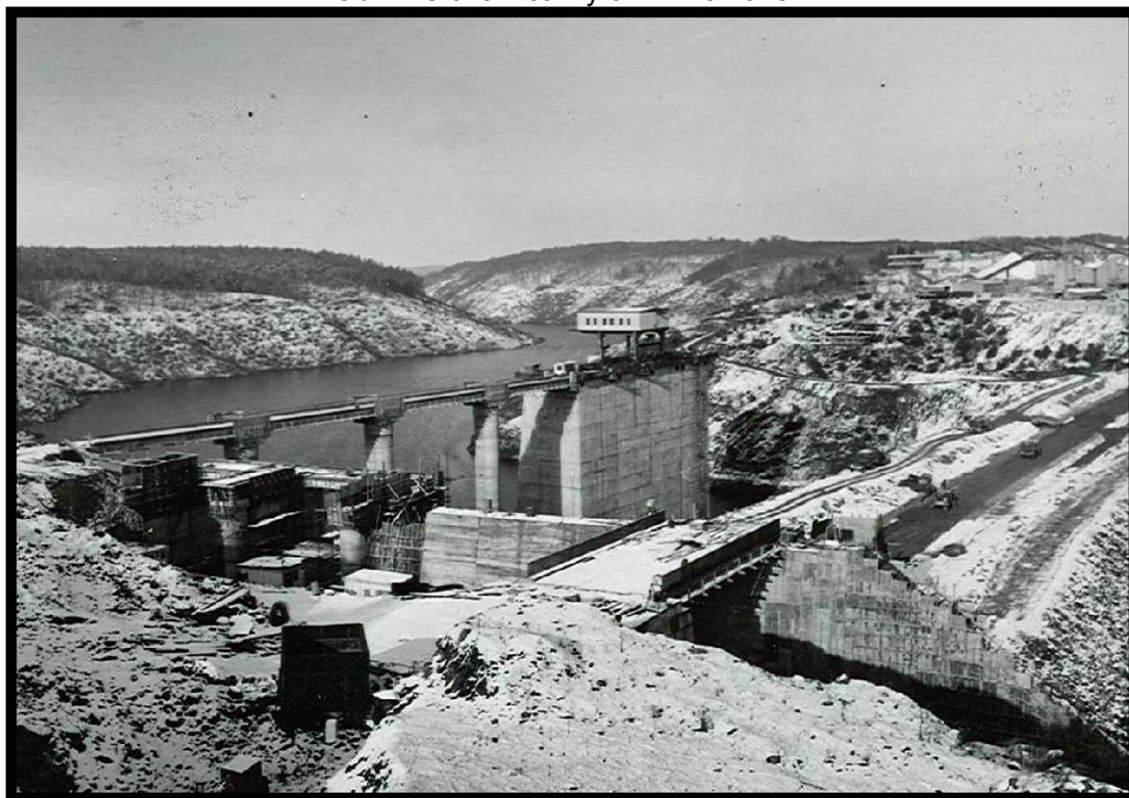
Stav napouštění hlavní hráze - 25.11.1976
