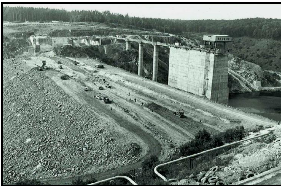
Obr. 3 Sypání hráze Kramolín – 12.9.1976
