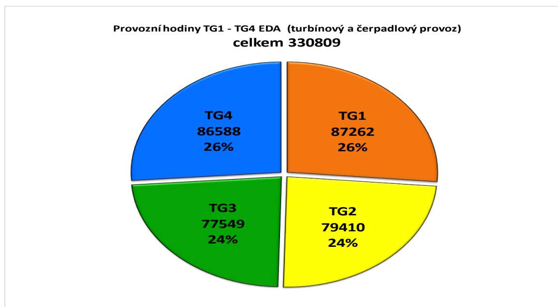
Graf 2 Provozní hodiny od uvedení do provozu do první poloviny roku 2018 [6]
