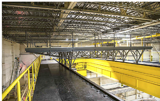
Zodolňování stropu reaktorovny je prováděno ze speciální plošiny umístěné na jeřábech Foto Jan Sucharda
