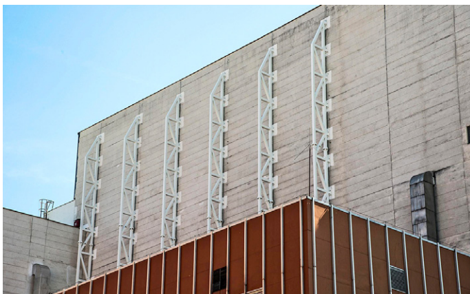
Západní štítová stěna reaktorovny (HVB I) s již provedeným zpevněním ocelovými žebry
